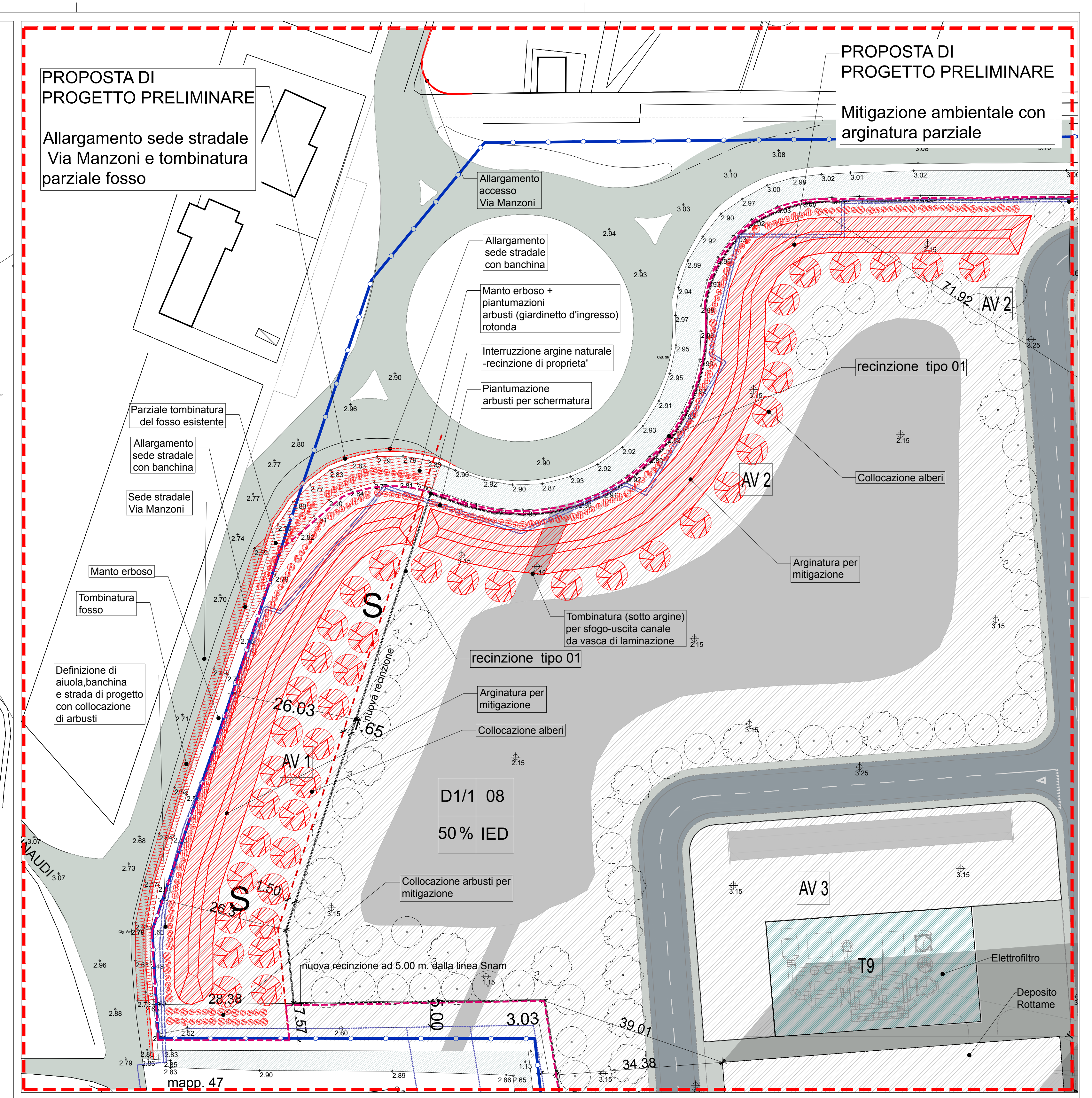
Planimetria generale - PLANIMETRIA DI PROGETTO PRELIMINARE_Area Nord - Ovest Asse stradale Via Manzoni scala 1 :500
