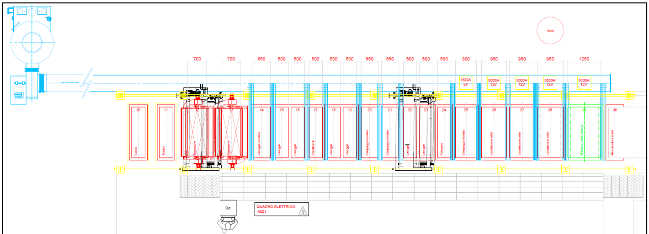
Figura 12. Layout nuovo impianto di elettrolucidatura.
